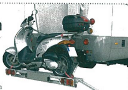
Movera-Heckträger mit 170 Kilo Traglast, 60 Kilo Gewicht.
